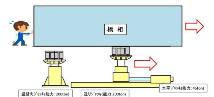
【橋脚上のジャッキ設備】
