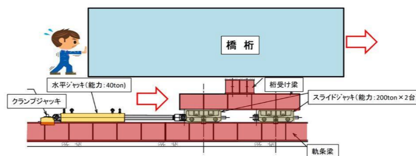
【陸上部のジャッキ設備】
