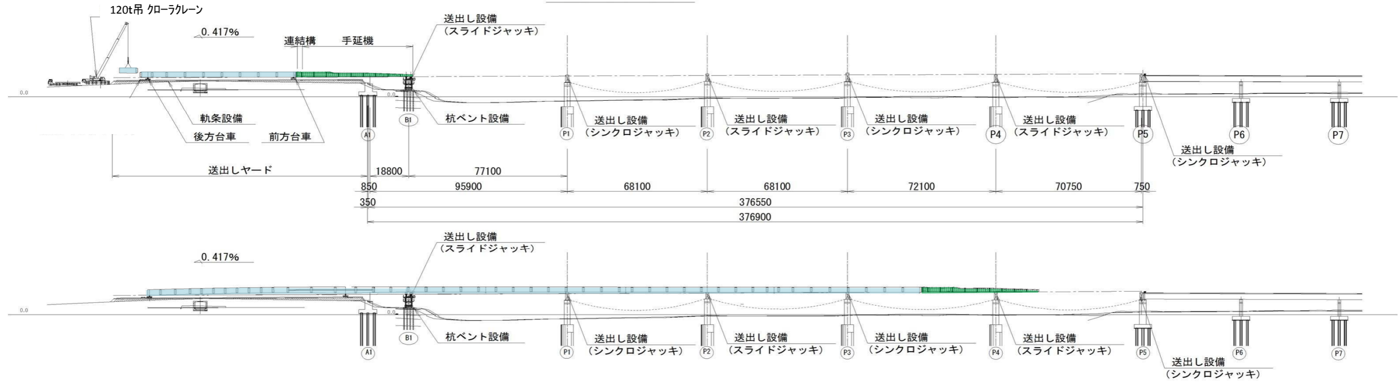
側面図
